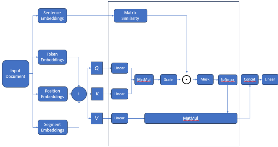
Hình 4.3. Bổ sung (chèn) tri thức cho BERT
