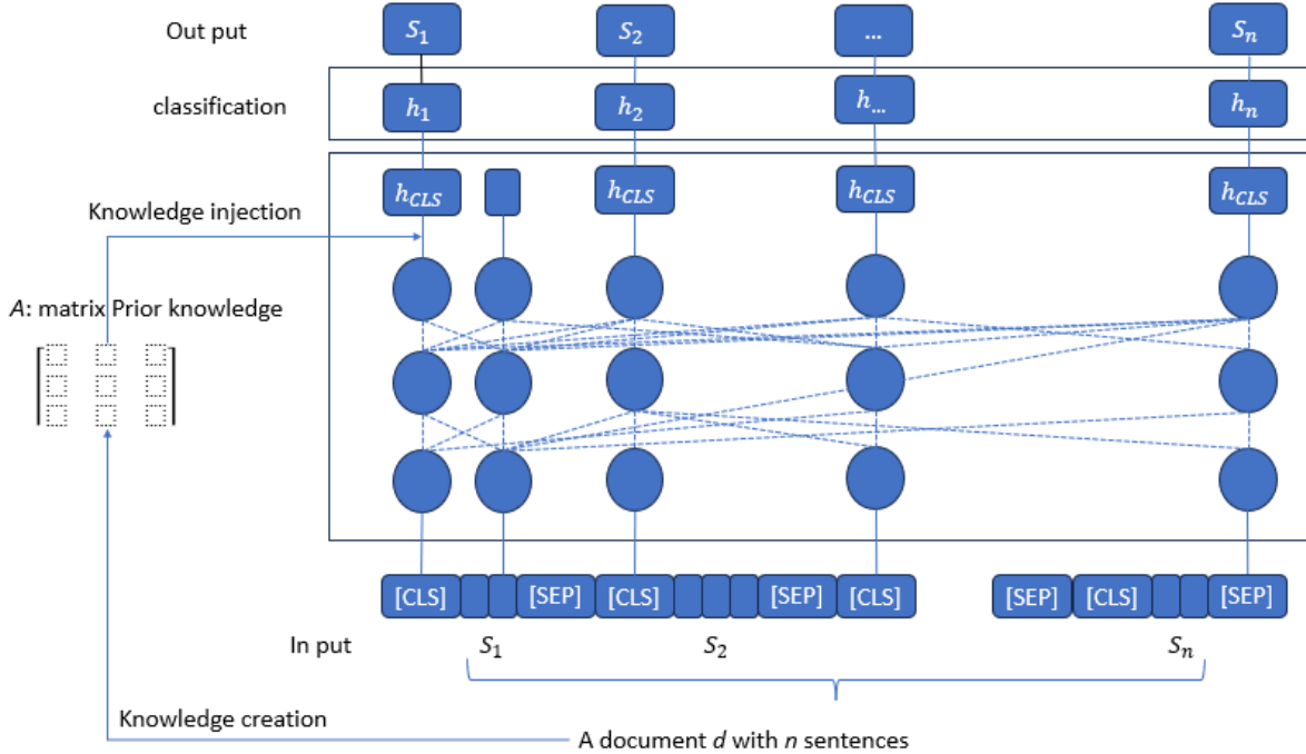
Hình 4.2. Mô hình BERT tóm tắt văn bản sử dụng tri thức nội tại
