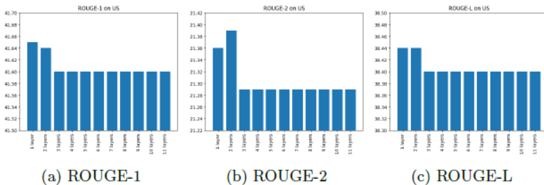
Hình 4.6. Tri thức được bổ sung từ LexRank vào US BillSum.
