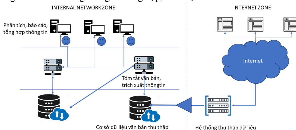
Hình 2.2. Hệ thống thu thập, phân tích và xử lý thông tin trên mạng Internet.
